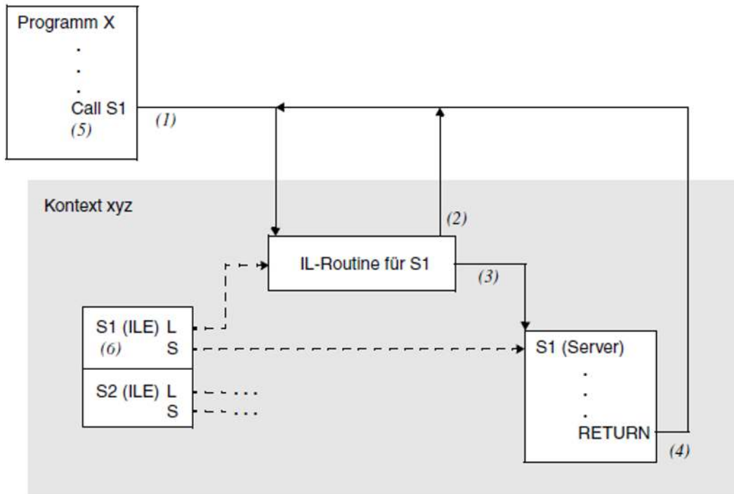
Bild 3: Indirektes Binden
