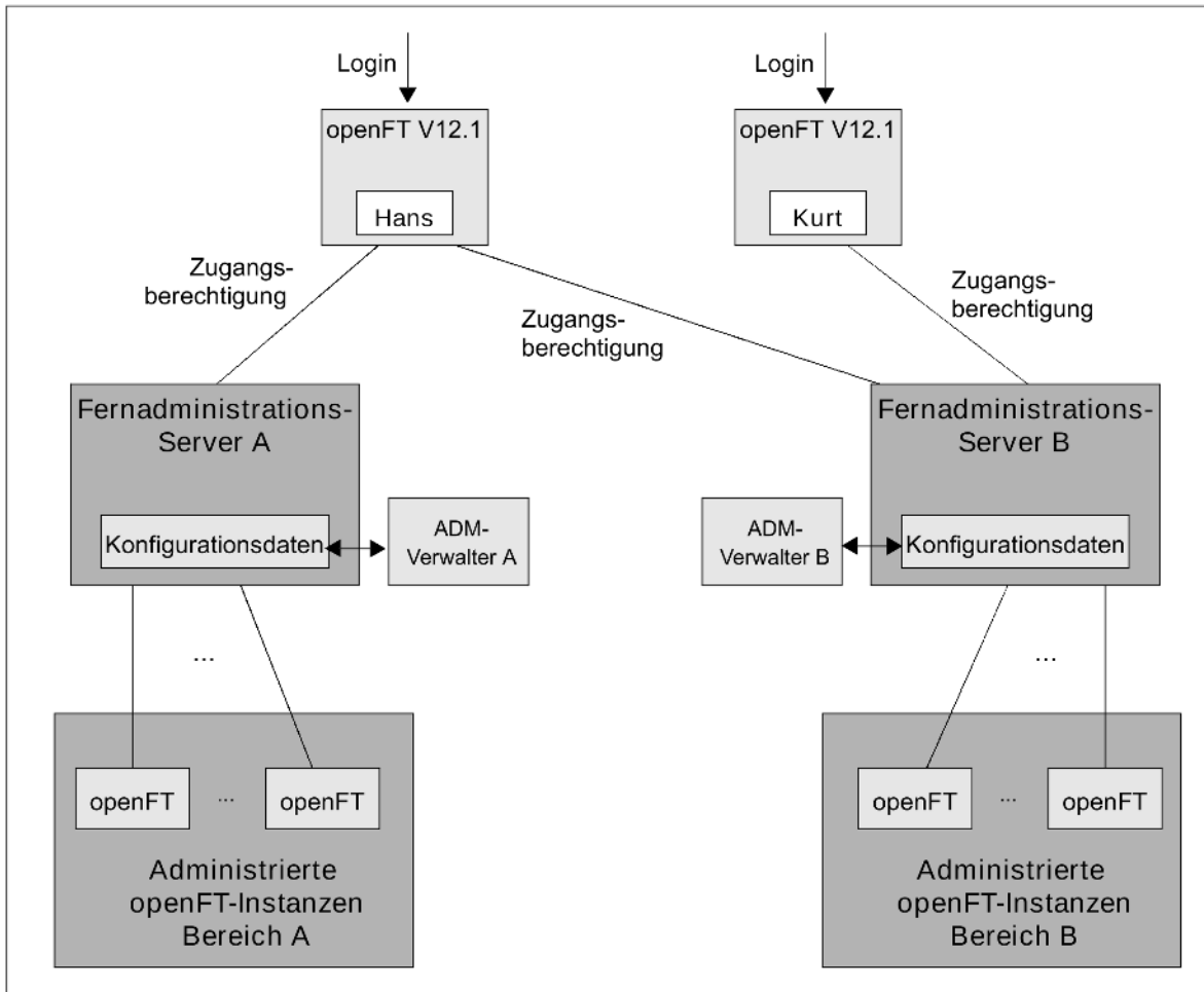
Getrennte Konfigurationen mit zwei Fernadministrations-Servern
