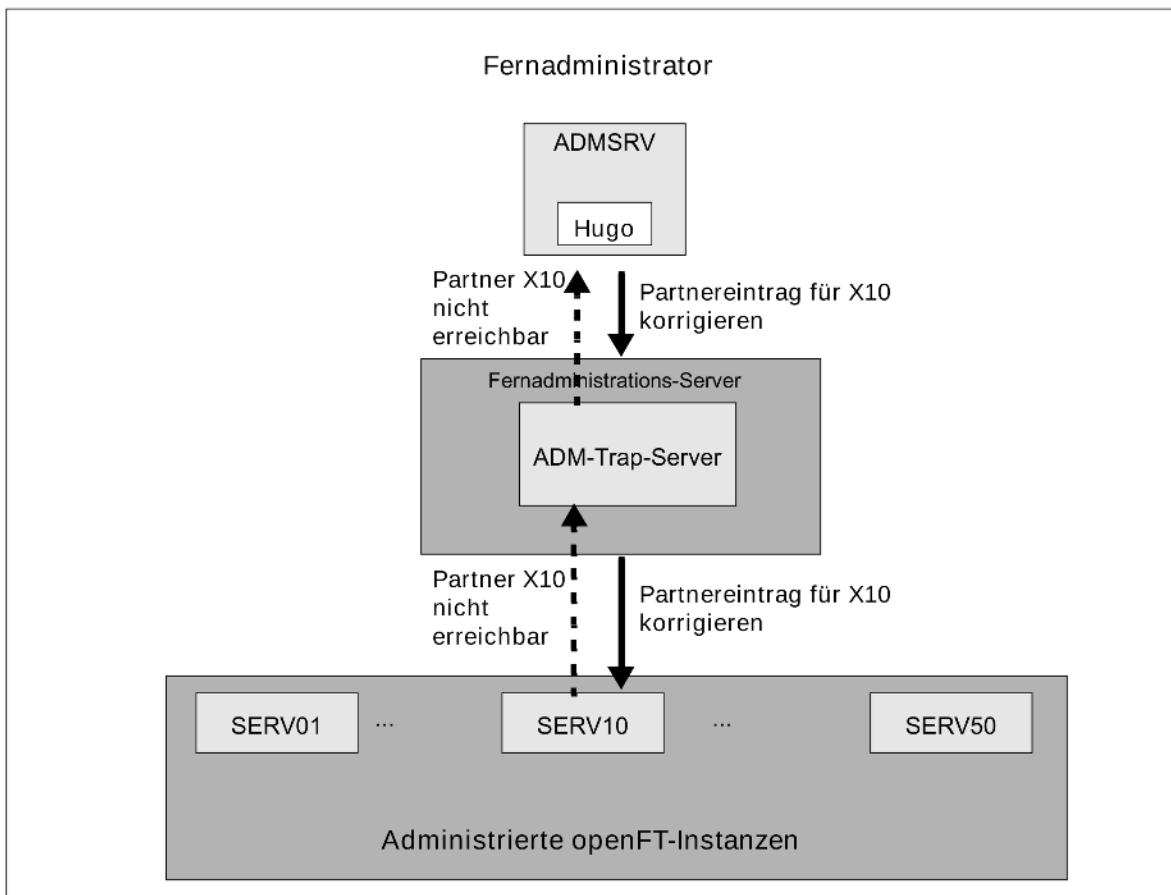
ADM-Trap-Server auf dem Fernadministrations-Server
