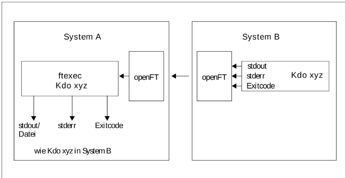
openFT-Konzept für ferne Kommandoausführung
