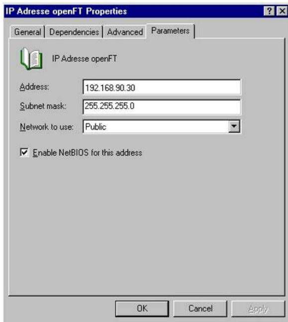
openFT im Cluster konfigurieren: IP Address - Parameters
