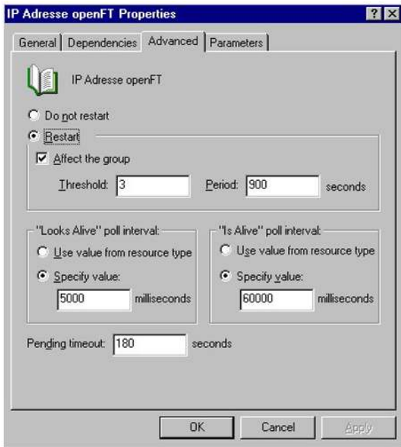
openFT im Cluster konfigurieren: IP Address - Advanced
